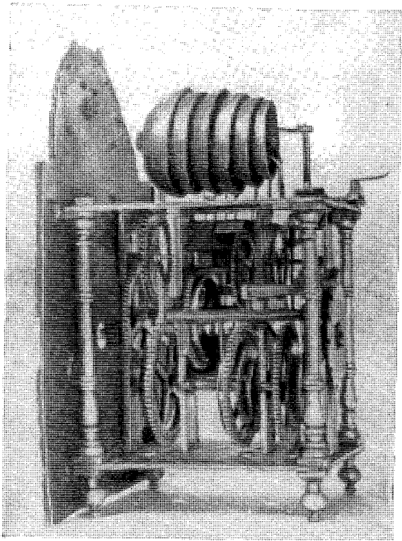
Рис. 10. Механизм настольных часов Петра Макарова
