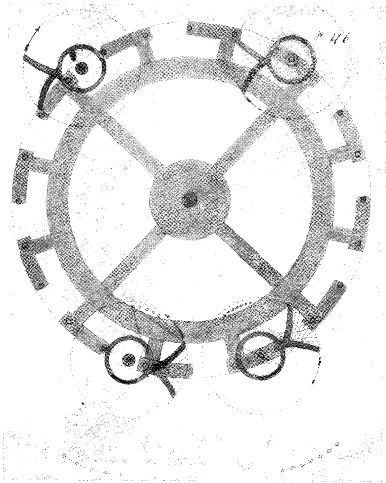
Рис. 19. Горизонтальный ход карманных часов И. П. Кулибина
