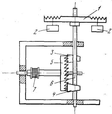
Рис. 2. Шпиндельный спуск с регулятором фоллио
