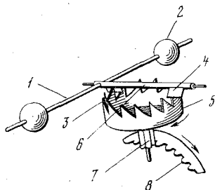
Рис. 2. Шпиндельный спуск с регулятором фоллио
