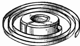
Фиг. 163. Правильная заштифтовка спирали.
