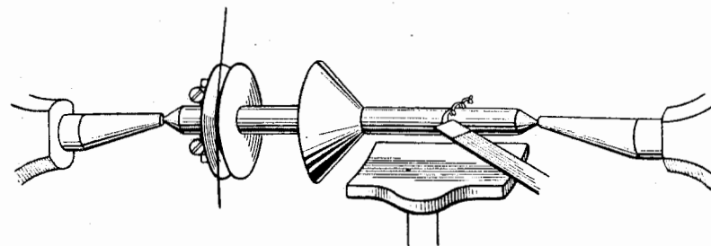
Фиг. 238. Обточка детали штихелем, установленным под углом.
