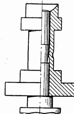
Фиг. 323. Положение выточки для крепления минутного триба.
