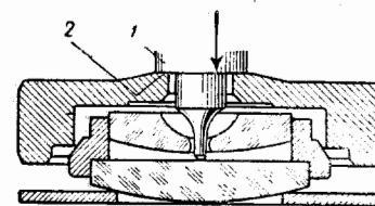
Фиг. 414. Действие осевого удара на запяток оси 1, упирающийся в опору; 2 — гнездо амортизатора «Parechoc».
