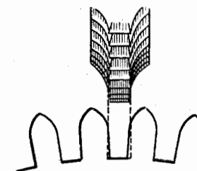
Фиг. 90. Латунная подставка для установки колеса. В вырезе колеса виден правильный диаметр подставки.
