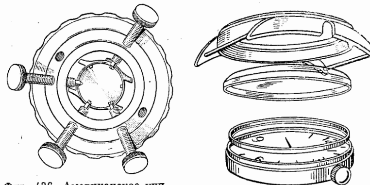
Фиг. 436. Американское универсальное приспособление «De Vries» для открывания корпусов.
