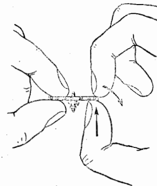
Фиг. 305. Правка обода не- разрезанного баланса.
