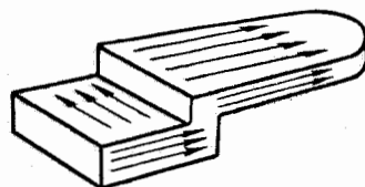
Фиг. 213. Направление штрихов при чистовой обработке моста баласа (показано стрелками).
