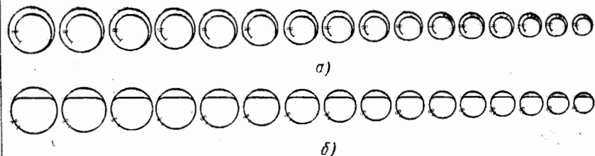
Фиг. 171. Концевые кривые спирали: а — концевые кривые Лоссье, б — концевые кривые Филлипса.
