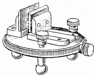
Фиг. 155. Приспособление для уравнивания баланса.
