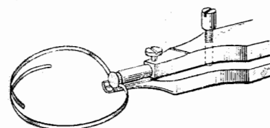
Фиг. 183. Специальный пинцет для изготовления концевой кривой.
