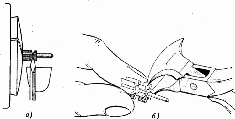
Фиг. 315. Отрезание лишней части триба: а — расположение штихеля при срезании только зубьев триба; б — удаление отрезанной части.
