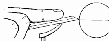
Фиг. 232. Неправильное расположение подручника — слишком далеко от обрабатываемой детали.
