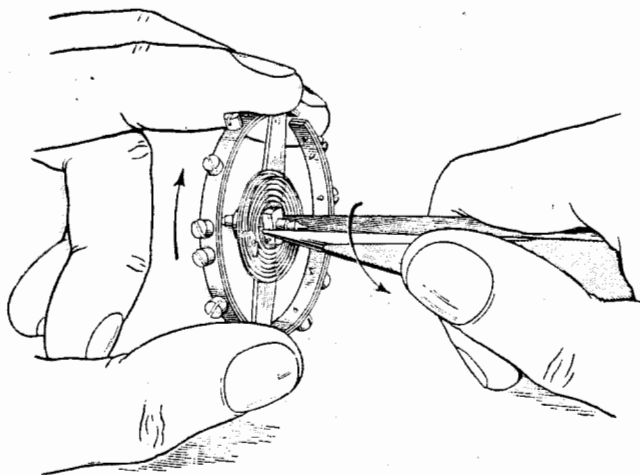
Фиг. 375. Съем колодки спирали.
