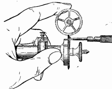
Фиг. 87. Способ держания колеса при подборе фрезы.
