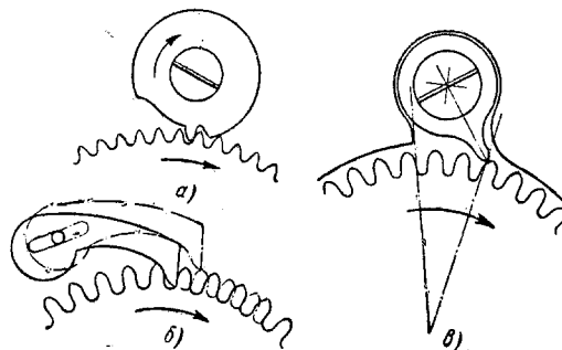
Фиг. 112. Собачки:
