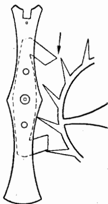
Фиг. 379. Ходовое колесо с храповыми зубьями: стрелкой показан зазор у затылка зуба для прохода палеты.
