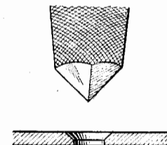
Фиг. 220. Инструмент для обработки отверстия под винт с потайной головкой.
