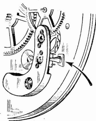
Фиг. 377. Анкерная вилка заклинена кусочками пробки.
