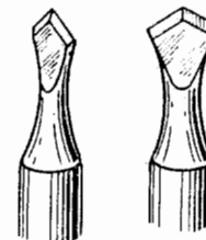
Фиг. 366. Форма сверла для сверления латуни.
