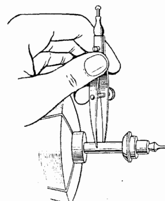
Фиг. 284. Кронциркуль для обмера трибов.
