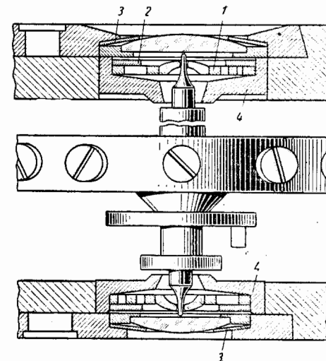
Фиг. 416. Противоударное устройство Shockresist:
