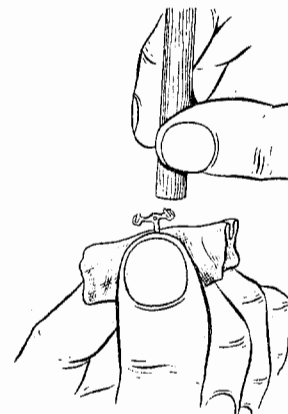
Фиг. 116. Способ чистки палет вилки.
