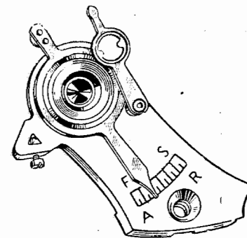
Фиг. 410. Амортизатор «Parechoc» с пружиной, допускающей смещение в одну сторону.
