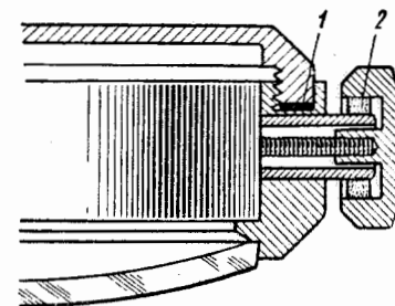
Фиг. 432. Сальниковая прокладка, вставленная в заводную головку:
