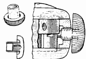
Фиг. 133. Втулка для устранения радиального зазора заводного вала.
