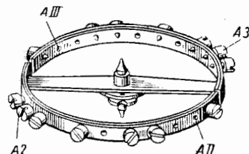
Фиг. 146. Дальнейшая температурная регулировка, выполняемая для того, чтобы часы спешили при высокой температуре. А2, А3, АII, АIII — отверстия для винтов.
