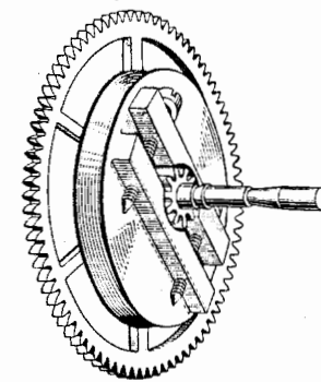
Фиг. 327. Оправка на колесе в рабочем положении.
