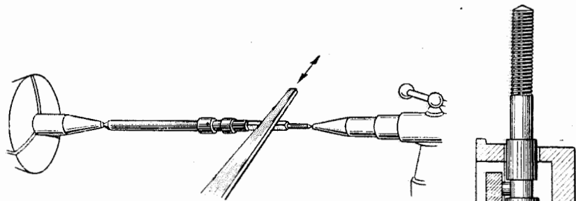
Фиг. 334. Свободное крепление вала между центрами; при полировке он самоустанавливается.
