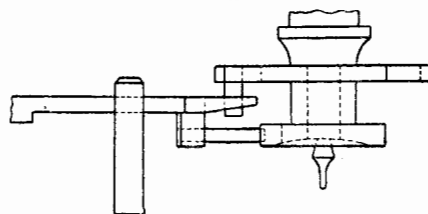
Фиг. 50. Правильное положение копы по отношению к предохранительному ролику.
