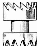
Фиг. 134. Увеличенный подрез зубьев (показаны пунктирными линиями).
