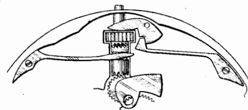
Фиг. 141. Зубья заводного триба застревают в зубьях кулачковой муфты.
