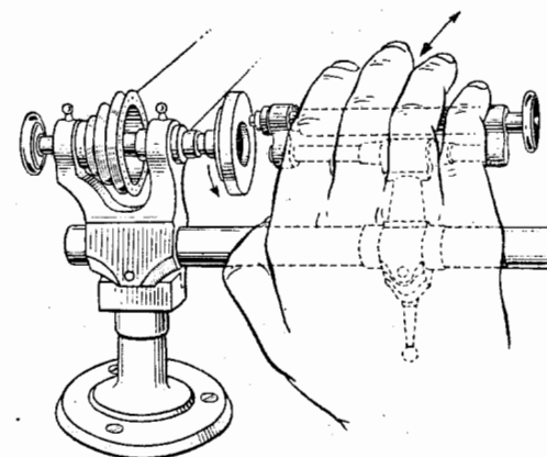
Фиг. 357. Ручная полировка головок винтов на станке.
