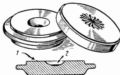
Фиг. 122. Масленка: 1 — капля масла; 2 — масло.
