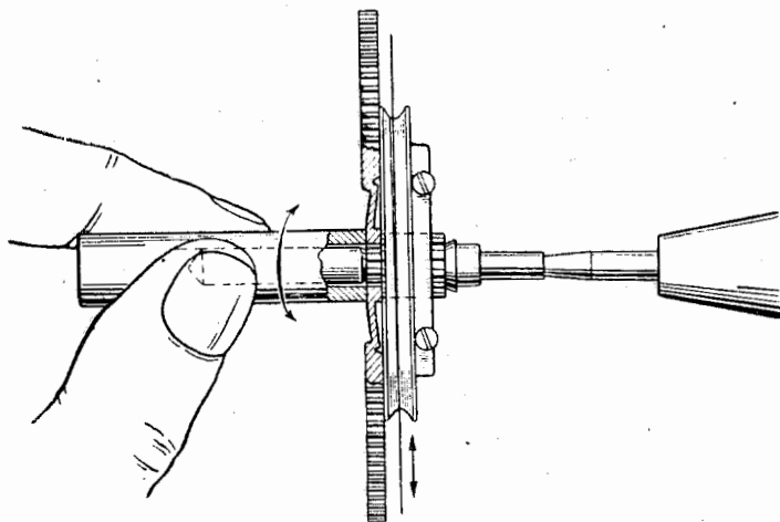
Фиг. 329. Обработка торца триба.
