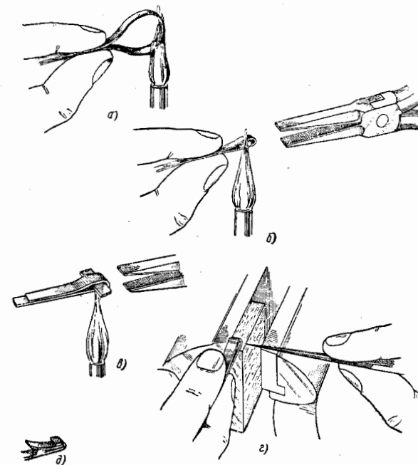
Фиг. 105. Изготовление крючка у заводной пружины: а — первый изгиб; б — второй более сильный изгиб; в — пружина при придании ей более острого изгиба; г — опилование для последующего излома; д — законченный замок.
