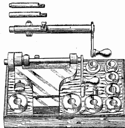
Фиг. 102. Приспособление для установки пружины в барабан американской конструкции.
