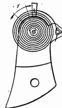
Фиг. 167. Наружный виток спирали на участке 1.
