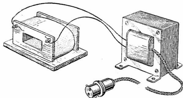
Фиг. 424. Катушка для размагничивания и присоединенный к ней трансформатор с вторичным напряжением 4, 6, 8 или 12 в (первичное напряжение соответствует напряжению сети питания).
