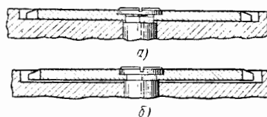
Фиг. 139. Заедание барабанного колеса. Запечник вала не проходит через платину; а — заклинивание; б — свободное перемещение.
