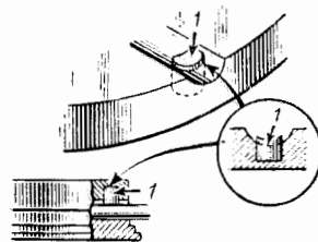
Фиг. 135. Забивание пробки в отверстие вала: 1 — пробка.
