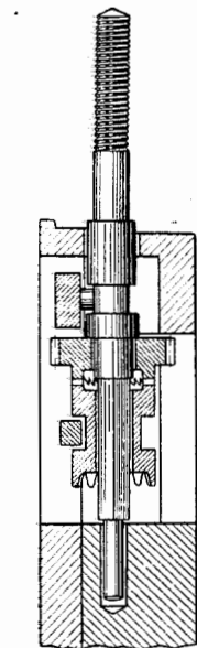
Фиг. 336. Вал, установленный в рабочем положении, следует обратить внимание на зазоры, на положение граней квадрата и выточки для штифта переводного рычага.
