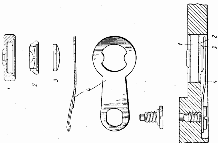
Фиг. 411. Амортизатор «Parechoc»; нижняя опора:
