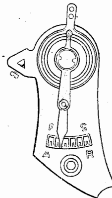
Фиг. 409. Амортизатор «Parechoc», отличающийся съёмной пружиной.
