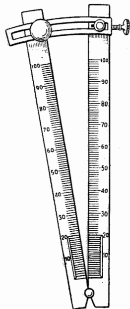
Фиг. 75. Сектор.
