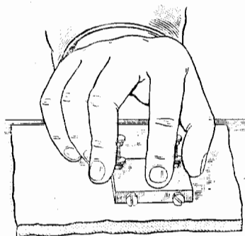
Фиг. 225. Способ применения приспособления с винтами.
