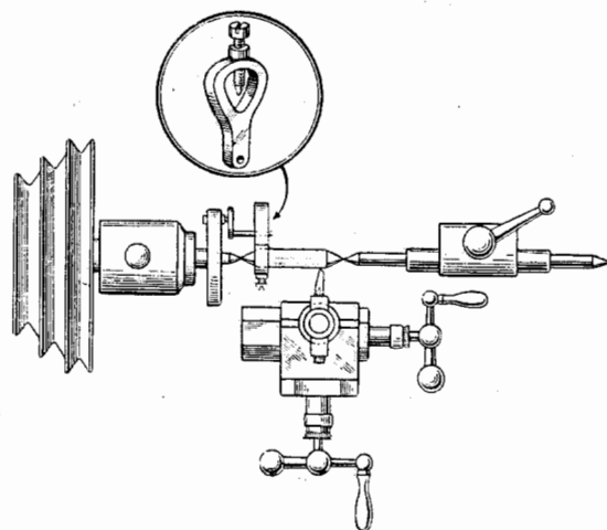
Фиг. 356. Обточка цилиндрических деталей с помощью суппорта.
