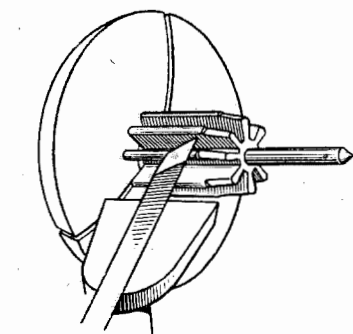
Фиг. 316. Обточка заплечика для посадки колеса.
