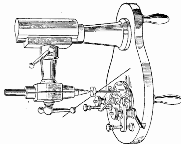
Фиг. 74. Рассверливание верхнего отверстия под ось секундного колеса.
