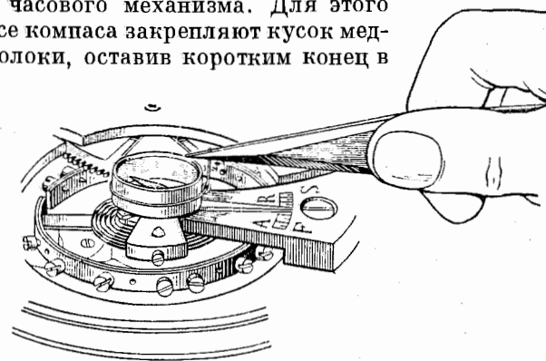
Фиг. 419. Испытание компасом намагниченности механизма часов.
