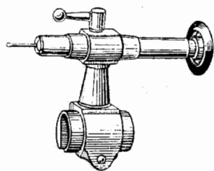
Фиг. 367. Сверло, закреп- ленное в задней бабке.
