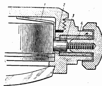
Фиг. 431. Заводная головка с уплотнительной втулкой:
