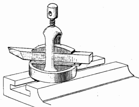
Фиг. 352. Регулировка высоты установки резца.
