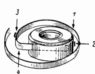
Фиг. 165. Регулировка положения внутреннего витка в колодке:
